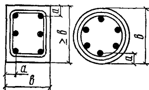
Рис. 1. Расстояния до оси арматуры
