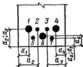
Рис. 2. Среднее расстояние до оси арматуры
