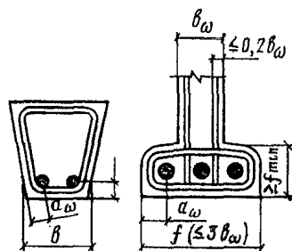
Рис. 3. Армирование балок и расстояния до оси арматуры
